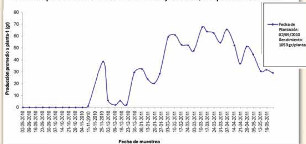
Curva de producción variedad Albion - Ensayo Batuco, temporada 2010 - 2011
